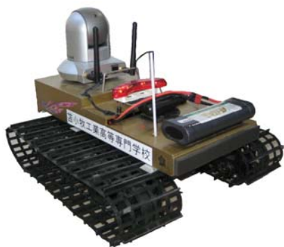
開発中カメラ付き小型ロボット
